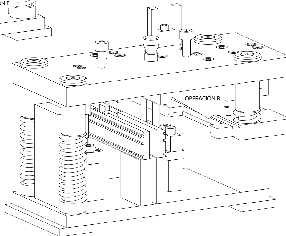
VISTA TRASERA
